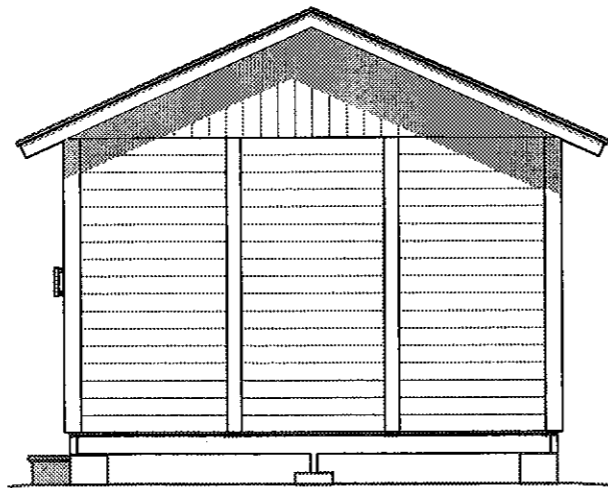
Julkisivut 1:50
